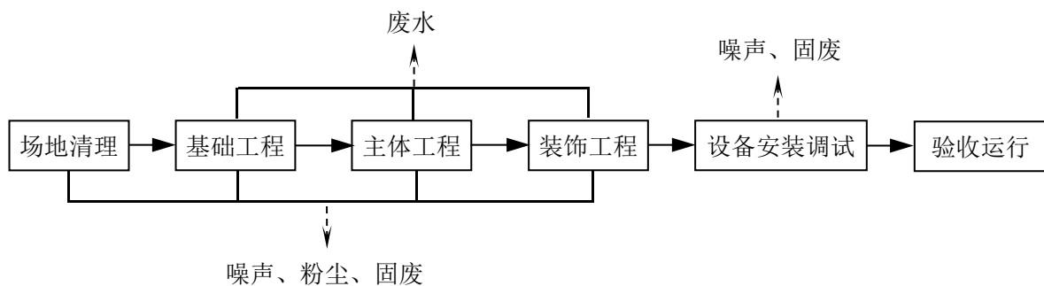
图 3.2-1 施工作业流程及产污环节示意图
