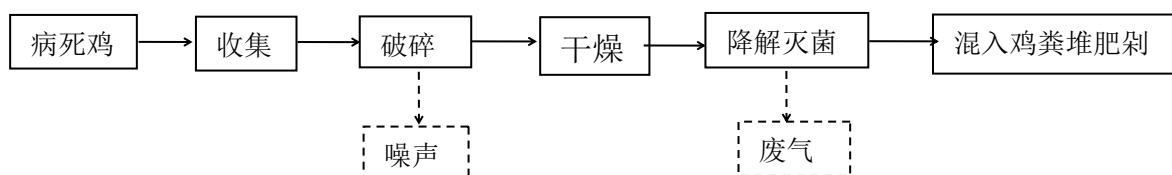
3.2-4 病死鸡无害化处理工艺及产污流程图
