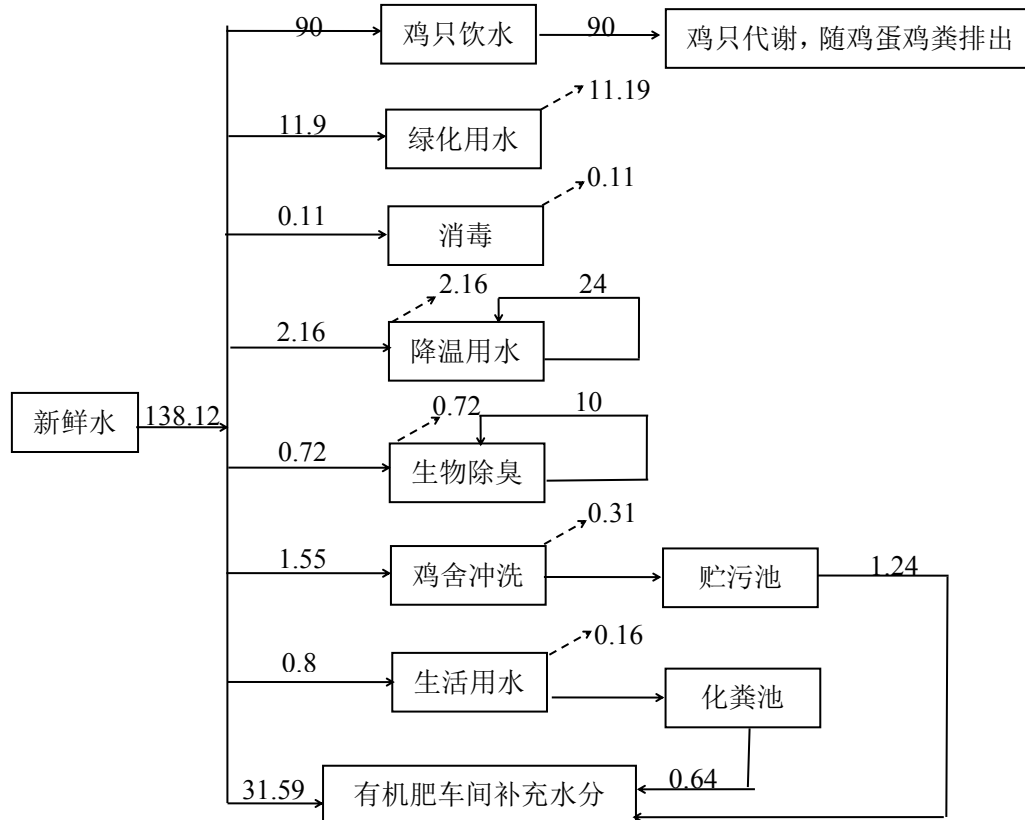
图 3.3-2 项目日最大水平衡图 单位 m³/d
