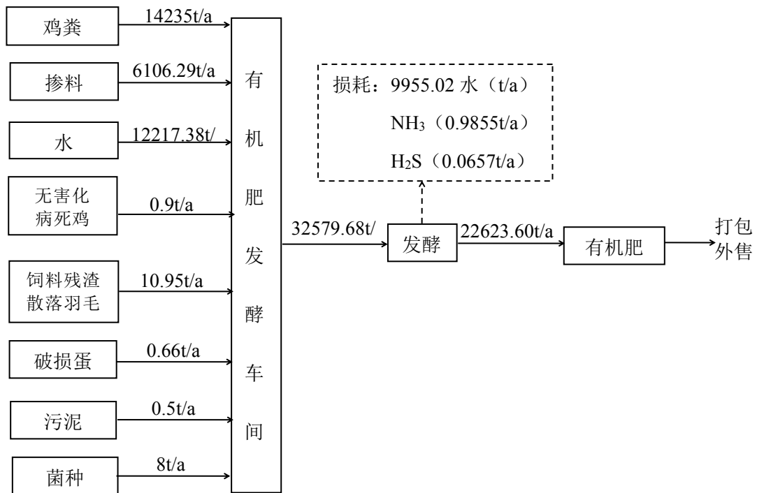
图 3.3-1 有机肥发酵车间物料平衡图 单位：t/a
