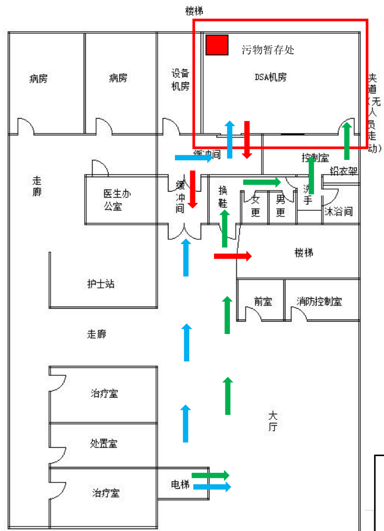
图 1-4 DSA 手术室楼层平面布局图及三通道图
