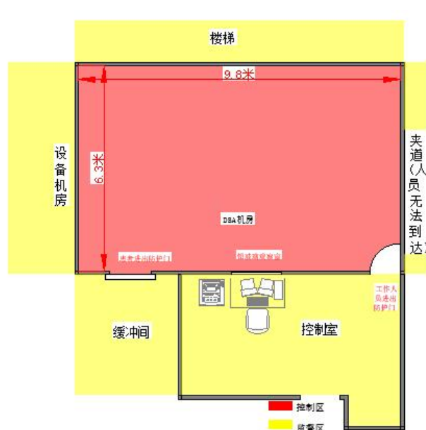
图 10-1 DSA 手术室工作场所分区管理示意图（平面）
