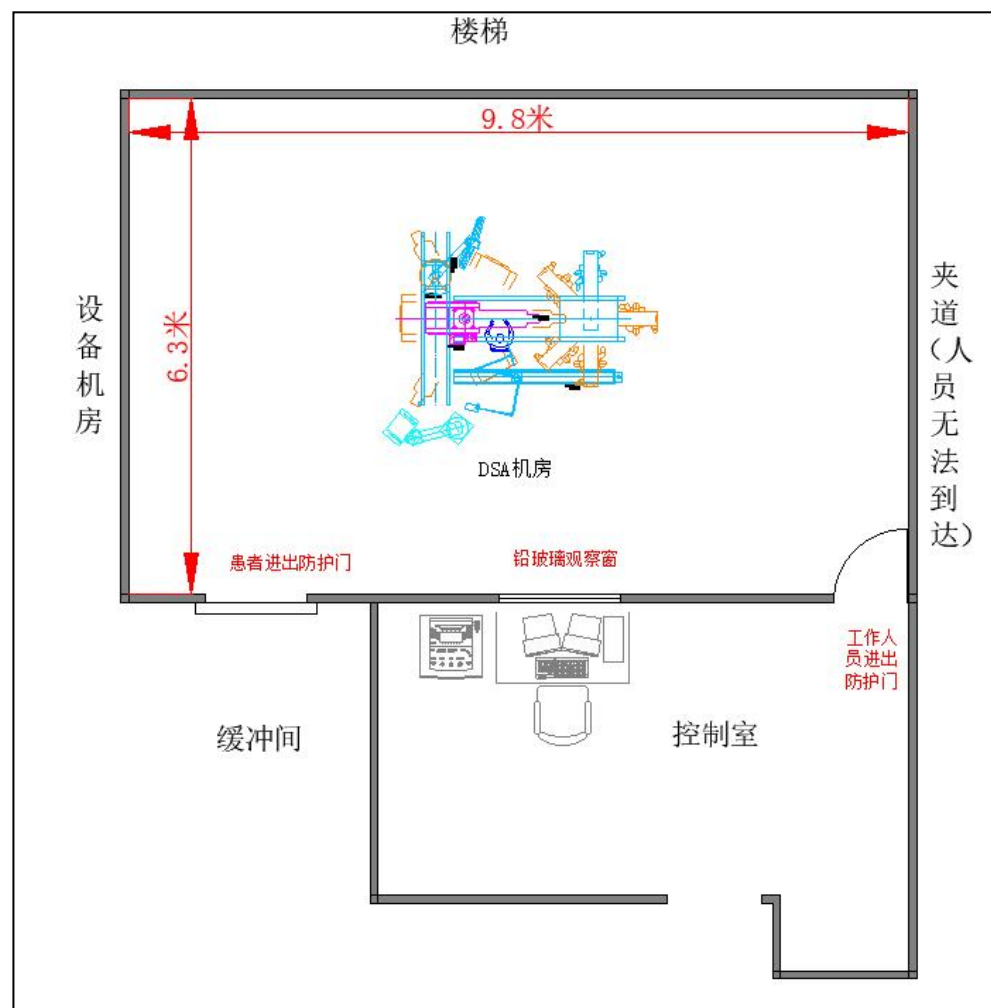
图 1-5 DSA 手术室平面布局图
