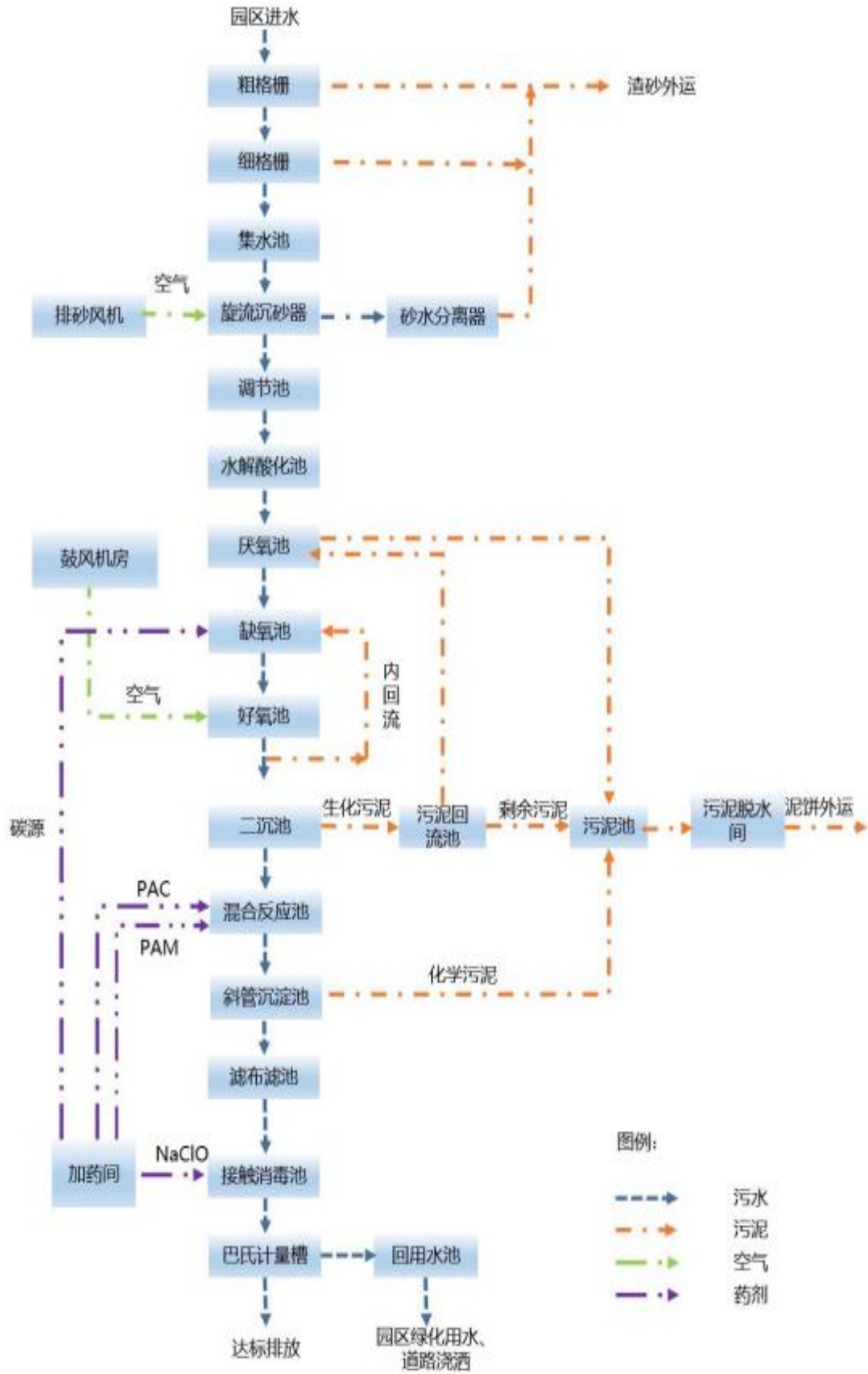
图 3.2-3 项目工艺流程图
