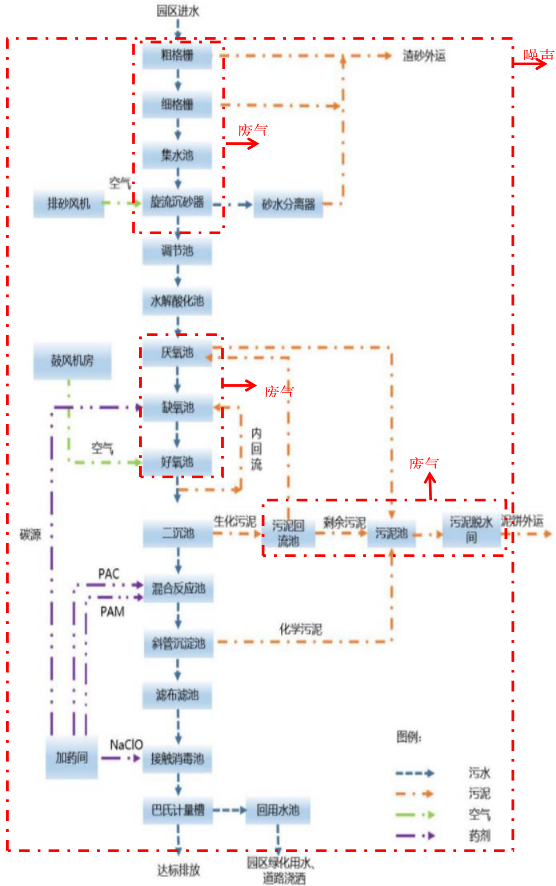
图 3.4-1 运营期工艺流程及产污环节图
