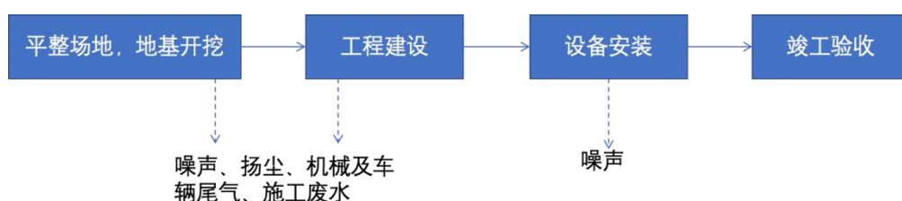
图 3.3-1 项目施工期工艺流程及产污环节图
