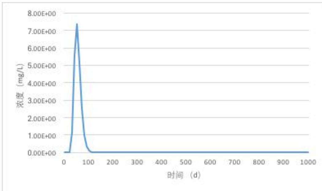
图6.3-2 发生非正常泄漏后下游厂界处浓度历时曲线
