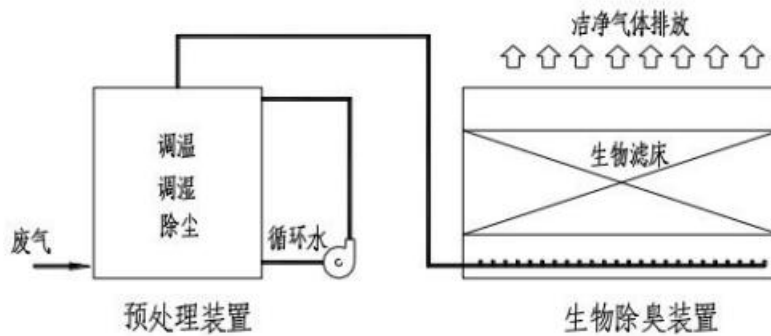
图 3.2-2 生物滤池除臭装置工艺流程图
