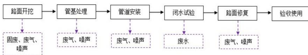
图 3.3-2 项目管道施工期工艺流程及产污环节图
