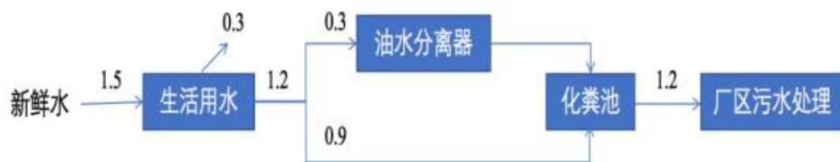
图 2.3-1 项目厂区用水水平衡图 单位：m 3 /d
