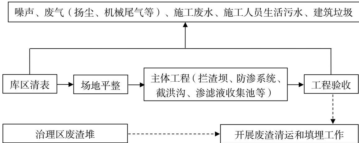
图 3-2 II类固废填埋场施工期工艺流程及产污情况图
