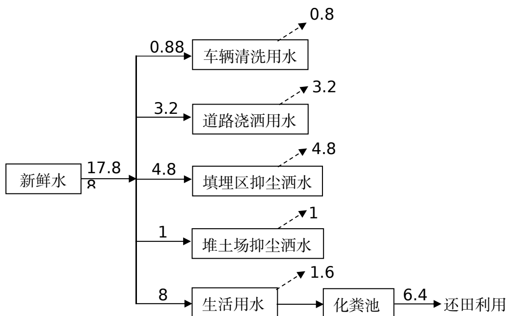
图 3-1 项目水平衡图 单位：m 3 /d
