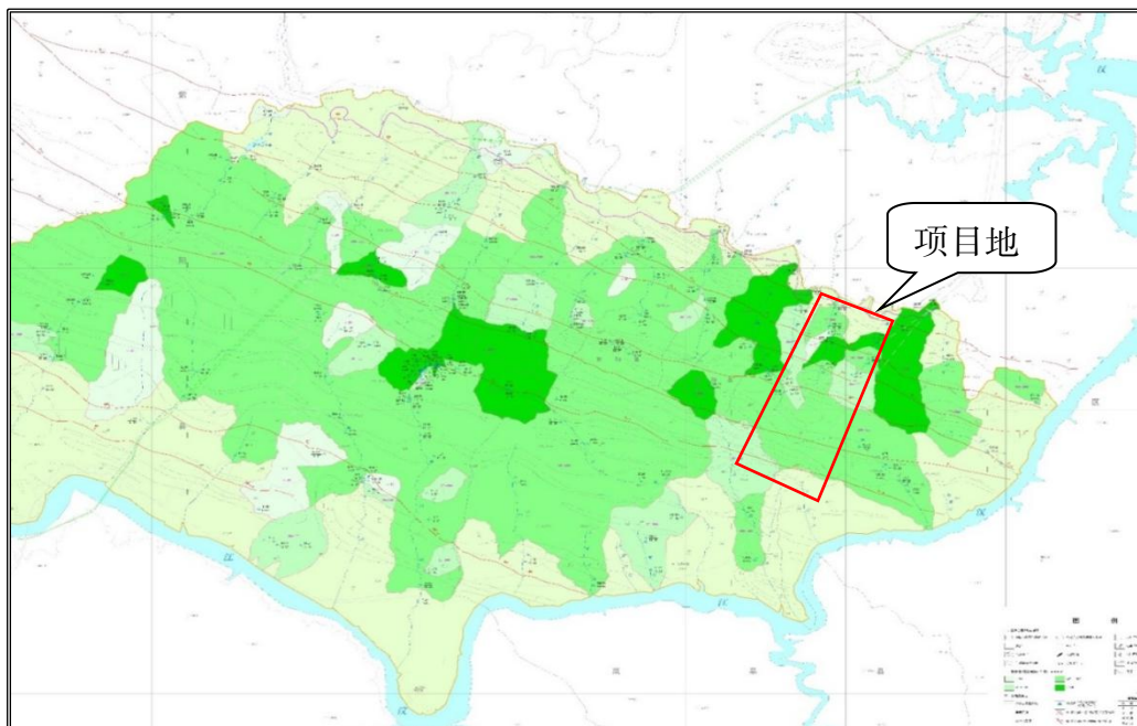
图 4.1 项目地水文地质图
