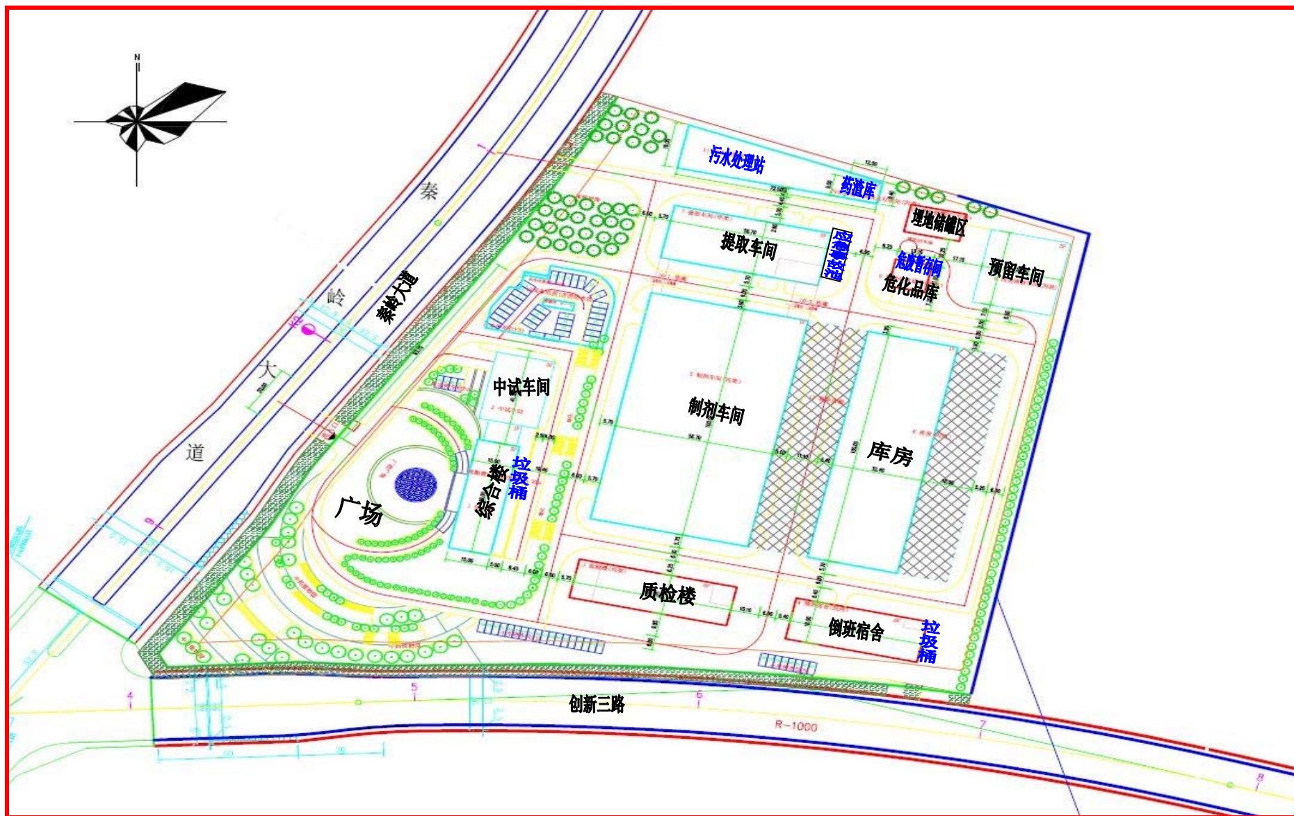
附图 3.2-2 厂区平面布置图
