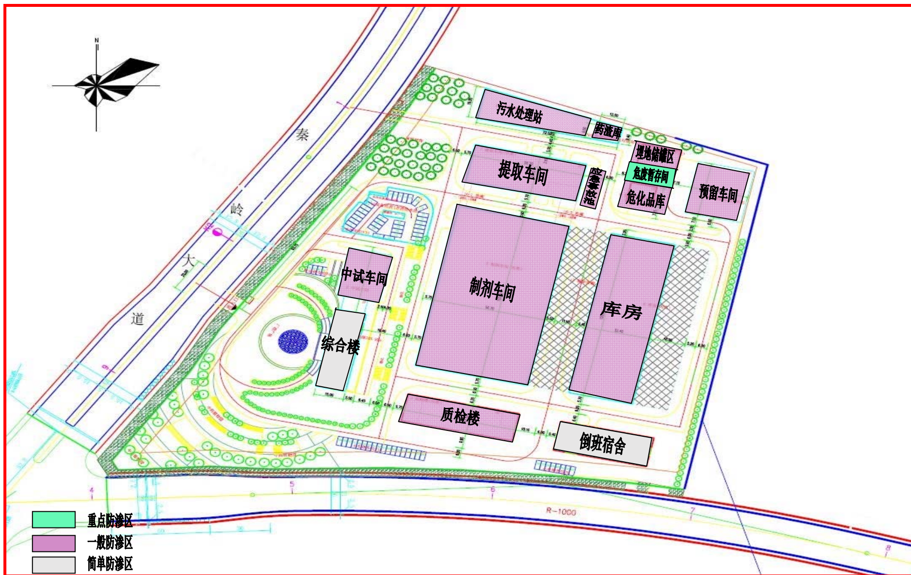
附图 6.3-1 厂区分区防渗示意图
